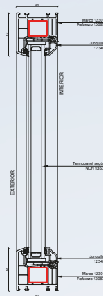
Detalle 2
