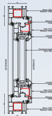
Detalle 1
